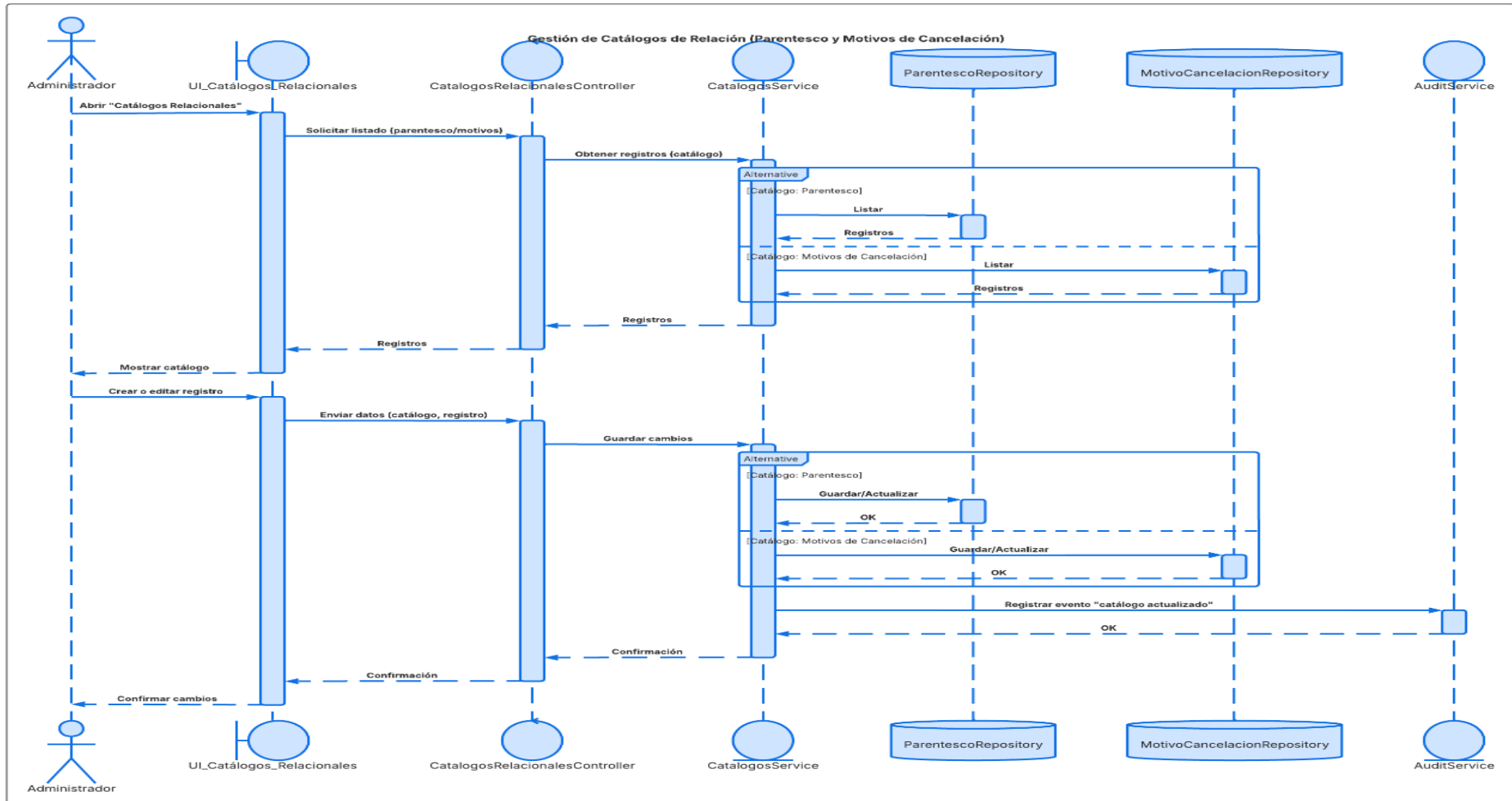
Ilustración 60 Secuencia Gestión de Catálogos de Relación
