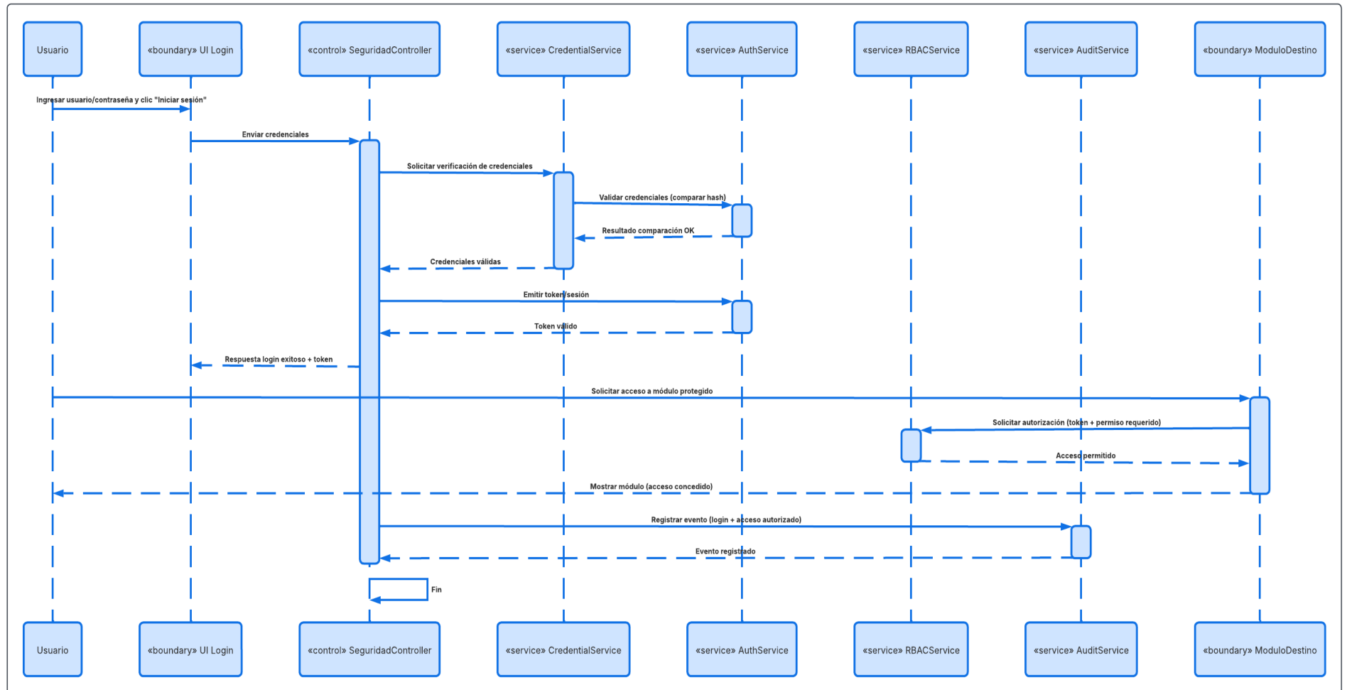
Ilustración 19 Secuencia Inicio de Sesión
