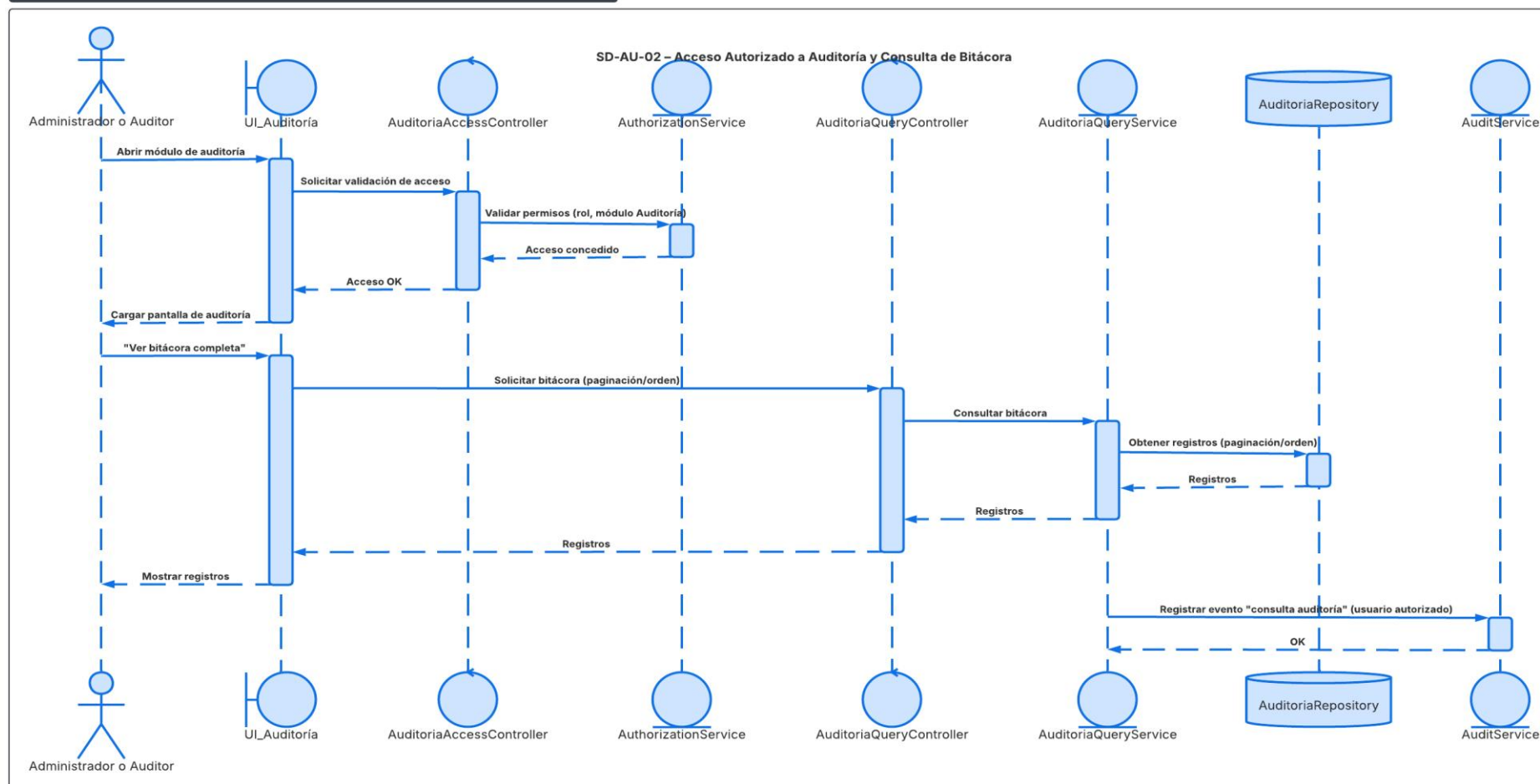
Ilustración 67 Secuencia Acceso Autorizado
