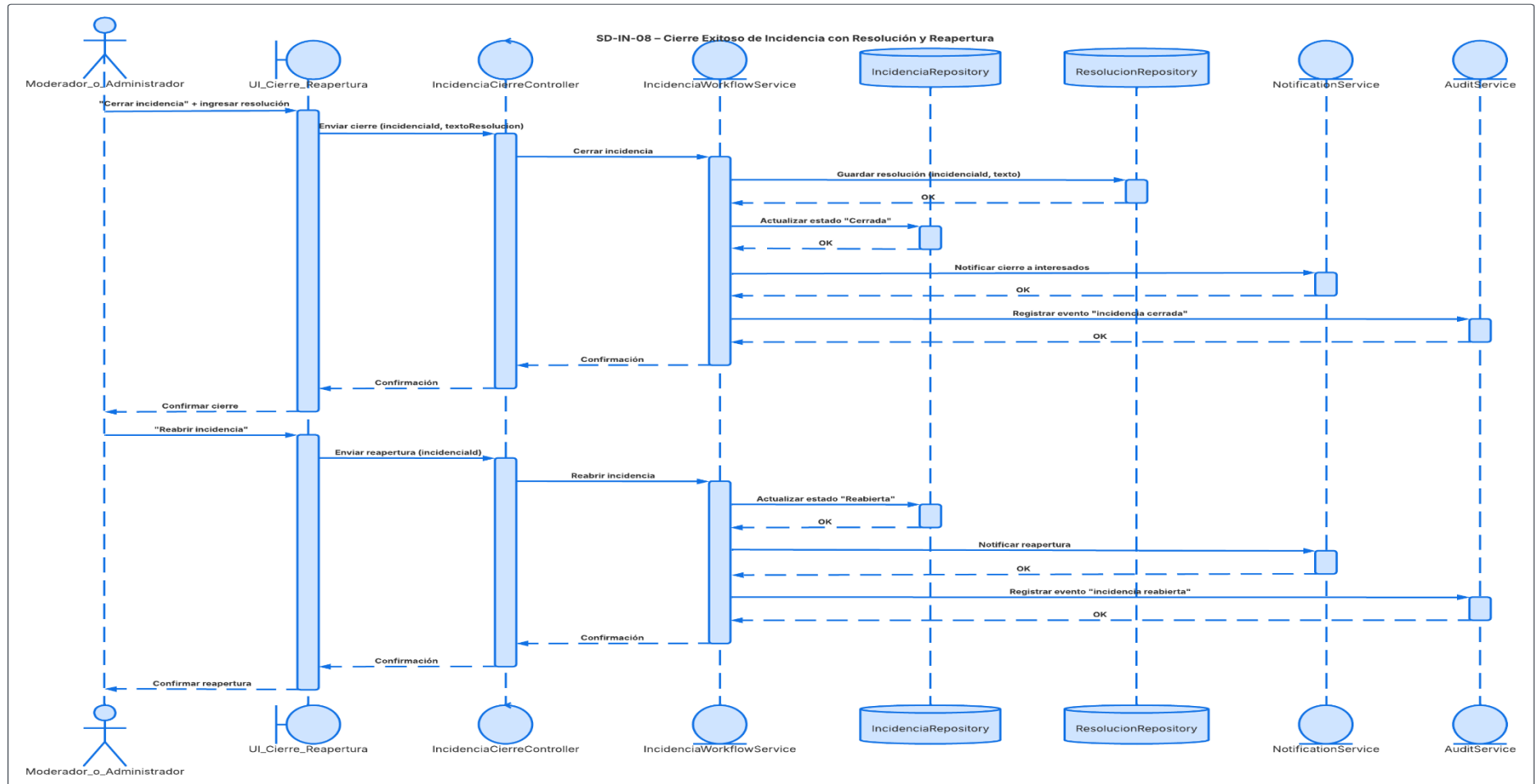
Ilustración 55 Secuencia Cierre de Incidentes
