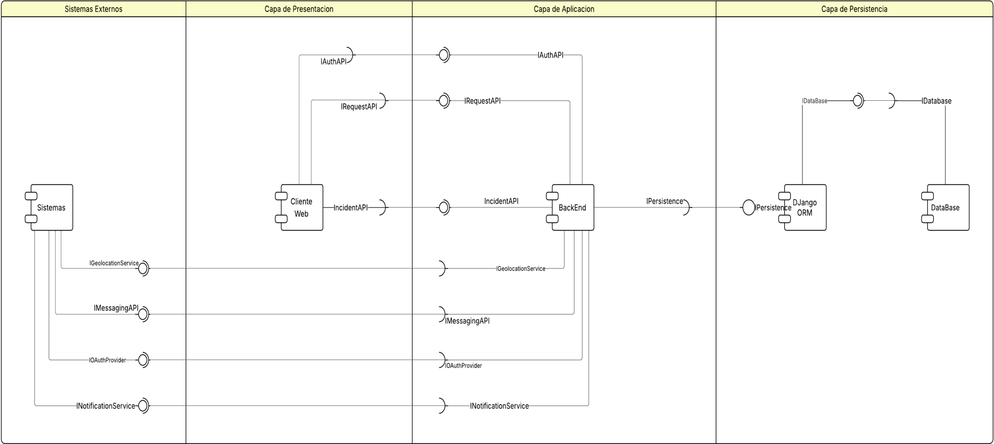
Diagrama de Componentes Barrio Solidario
