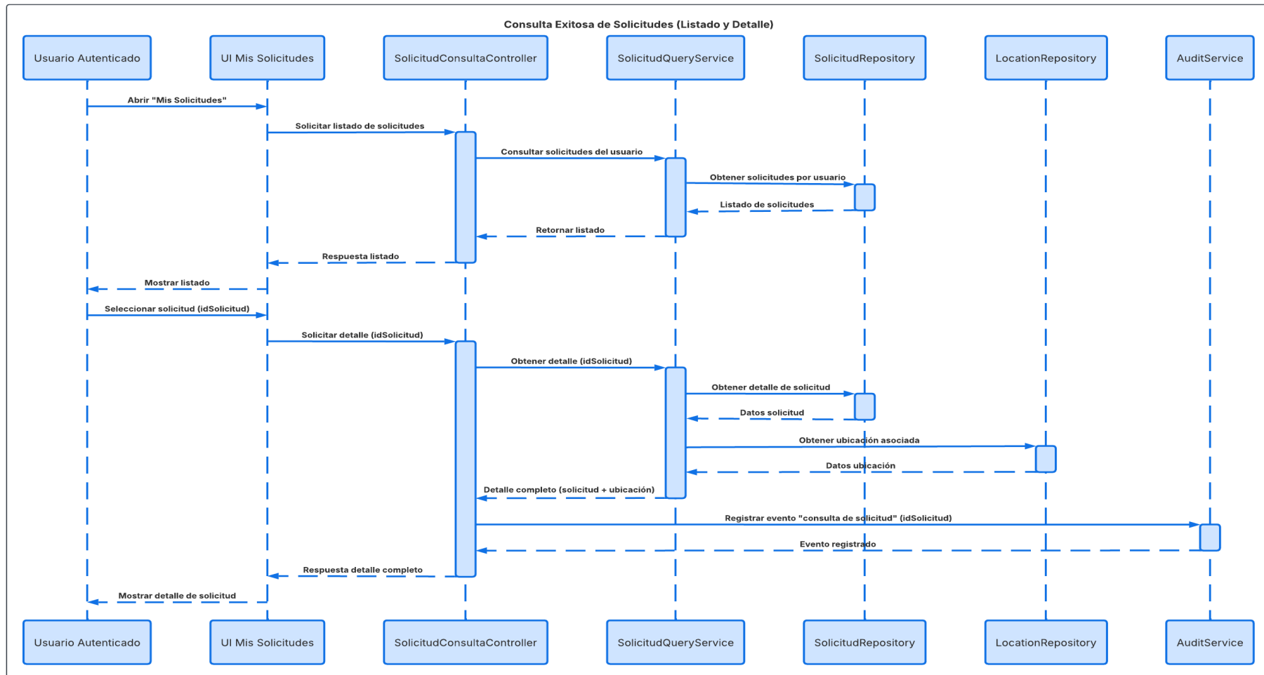
Ilustración 31 Secuencia Consulta de Solicitudes
